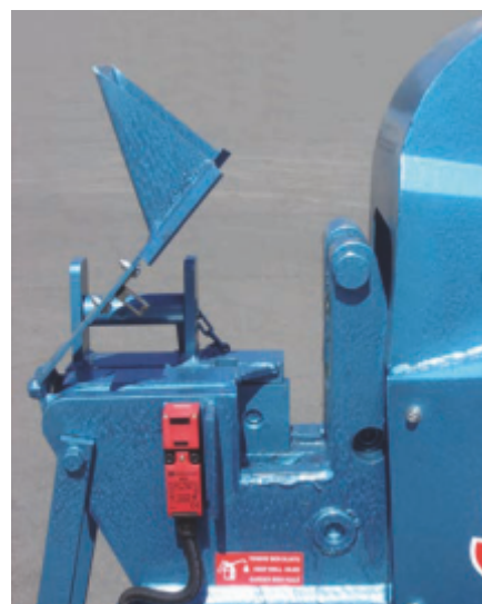
Grilaj protectie lama de taiere
